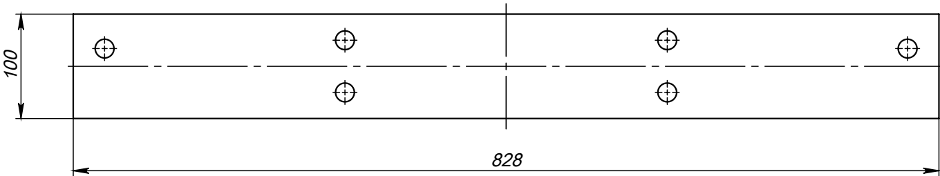
Поз.1 (Полухомут) развертка
