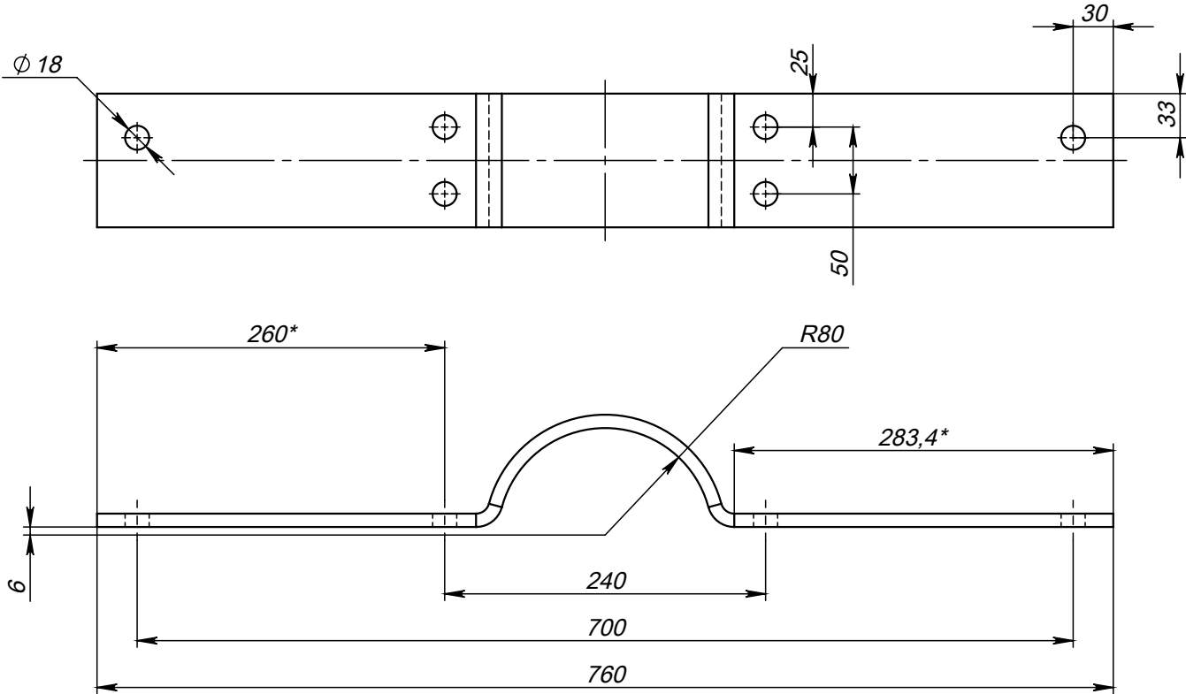
Поз.1 (Полухомут)
