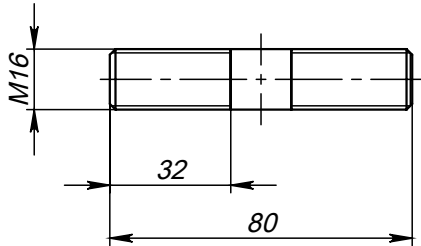
Поз.3 (Шпилька)
