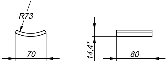
Поз.2 (Упор)
